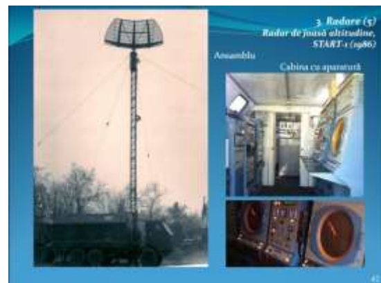
Primul radar românesc START-1
