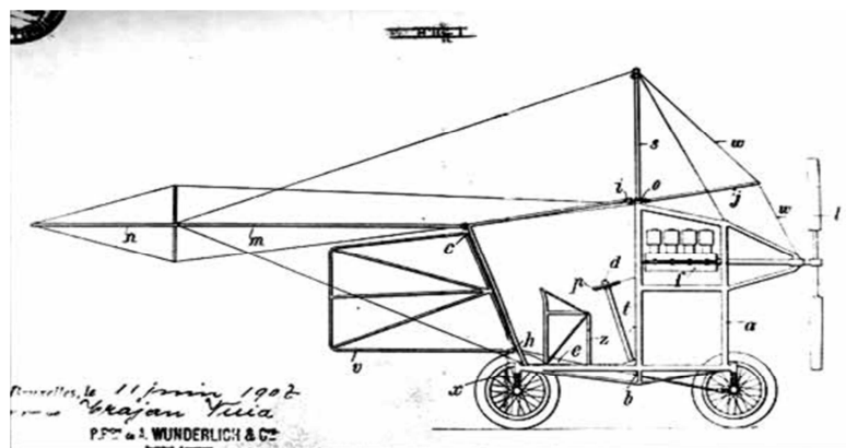
Schița privind avionul „Voia nr. 2”, brevetat la Bruxelles în Belgia, în anul 1907.
